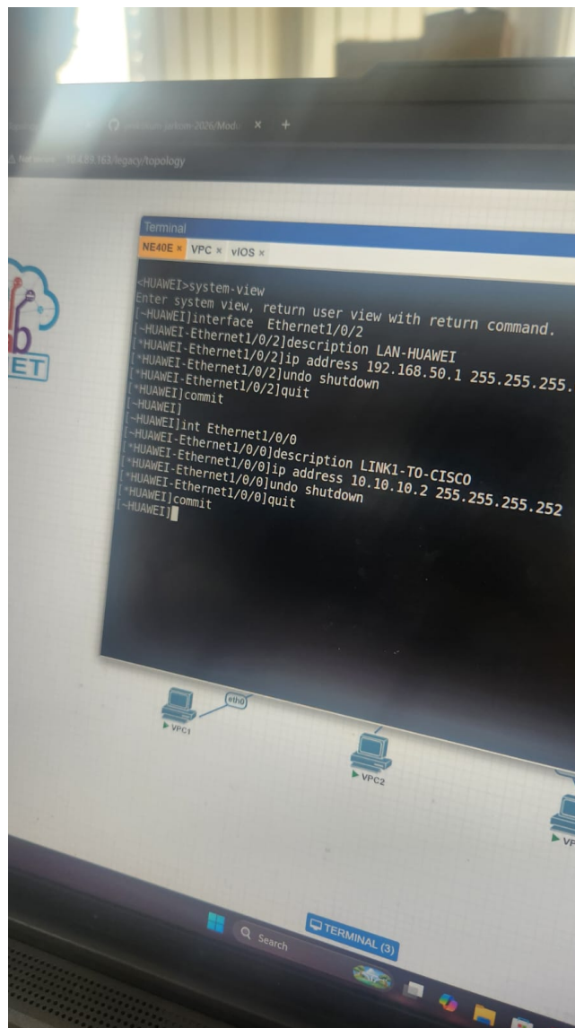
Gambar 10: Huawei ke lan dan ke cisco
