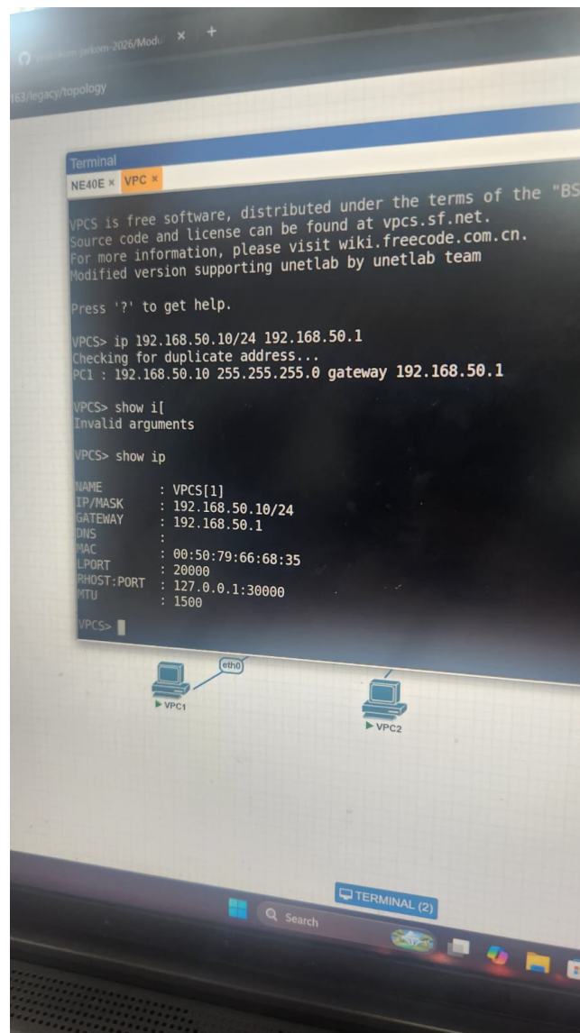
Gambar 12: Vpc lan huawei
